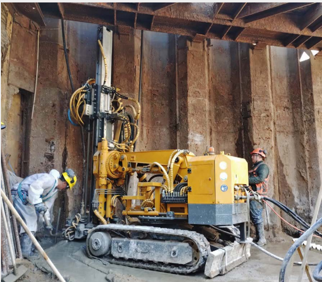
Einbau der Mikropfähle.
